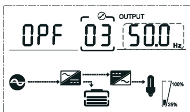
Настройка частоты
