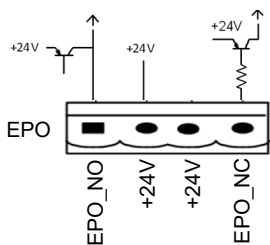
Рисунок 3.8. Схема входного порта для дистанционной подачи команды EPO
