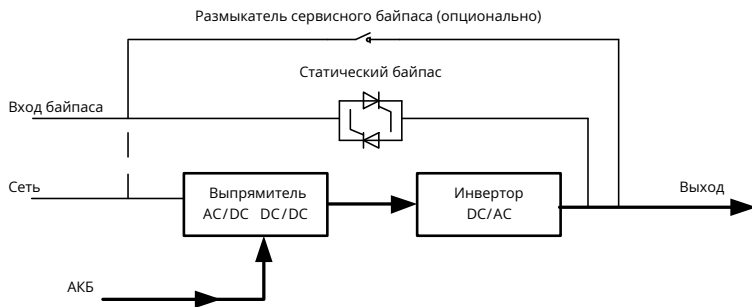
Рисунок 2.5. Функциональная схема ИБП при работе от АКБ
