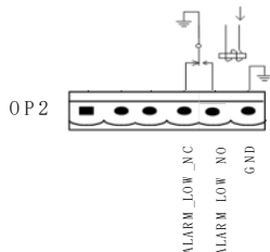
Рисунок 3.13. Схема интерфейса выходного релейного контакта общей тревоги
