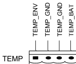
Рисунок 3.9. Порты TEMP 1-4 для определения температуры
