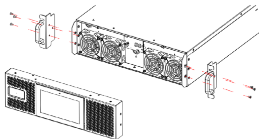
Рисунок 6.3. Демонтаж лицевой панели
