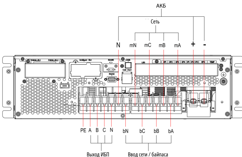
Рисунок 3.16. 3-фазный ввод, 3-фазный выход, раздельный ввод сети и байпаса
