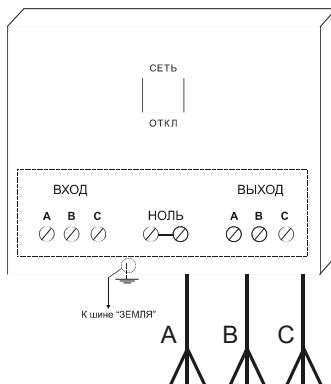
Рис.1 Вид блока коммутации со снятой крышкой
