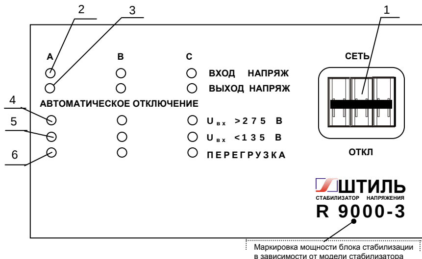
Рисунок 4.1 Передняя панель стабилизатора
